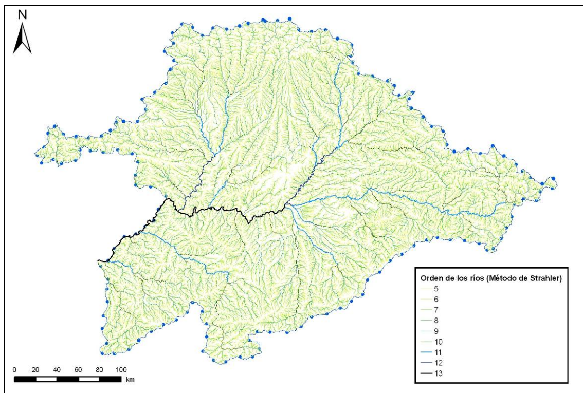
Figura 3. Órdenes Strahler
