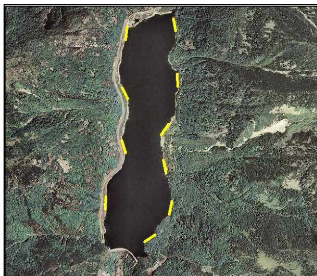
Figura 6 - Zonas de muestreo de helófitos en lagos con un perímetro mayor a 1 km
