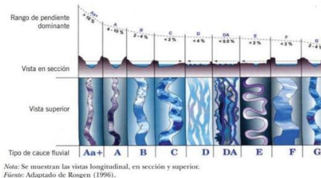
Figura 18.-Tipos morfológicos en planta para tramos no alterados según Rosgen (1996)
